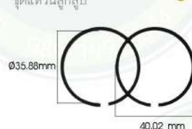
■ HG180-66 Ring set ชุดแหวนลูกสูบ
