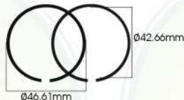
KM950-14 Piston ring แหวนลูกสูบ
