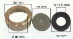
■ HG-CA-004 Spray gun head หัวพ่นยาทองเหลือง
