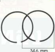
HG767-20 Piston ring แหวนลูกสูบ
