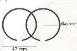
WP20-037 Piston ring set ชุดแหวนลูกสูบ
