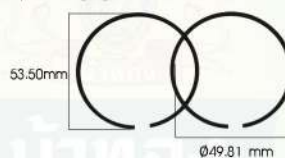
■ HG381-27 Piston ring set ชุดแหวนลูกสูบ
