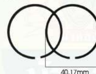
■ HG38-04 Ring set ชุดแหวนลูกสูบ
