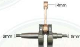
■ HG-44F-06 Crank shaft ชุดข้อเหวี่ยง
