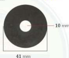
■ HG52-90 High pressure cap ฝาปิดแรงดัน
